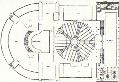
PLANTA CUARTO ANFITEATRO COTA + 13,80
