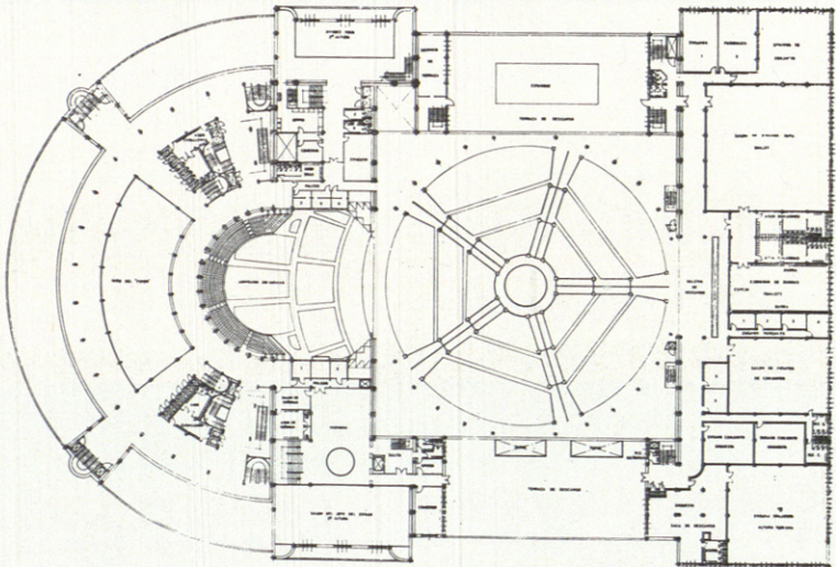
PLANTA SEGUNDO ANFITEATRO COTA + 7,80
