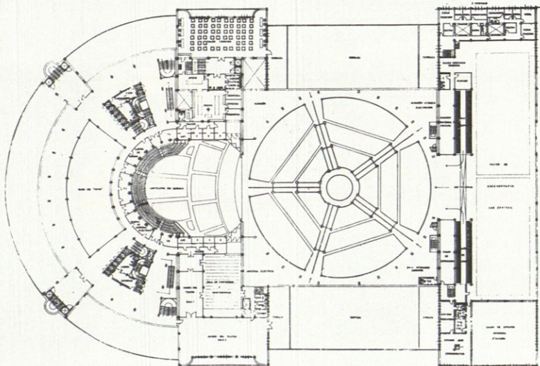
PLANTA TERCER ANFITEATRO COTA + 10,80
