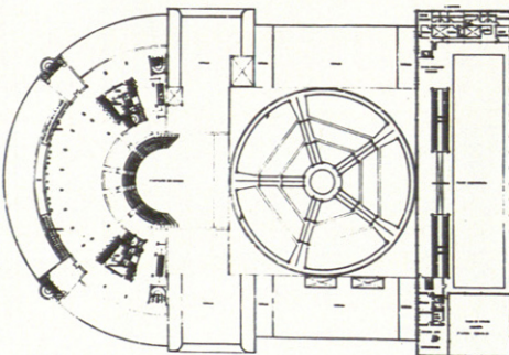
PLANTA QUINTO ANFITEATRO COTA + 16,80
