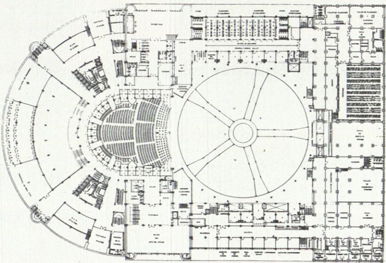
PLANTA PRIMER ANFITEATRO COTA + 4,80
